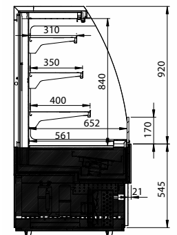
SEZIONE C-C
